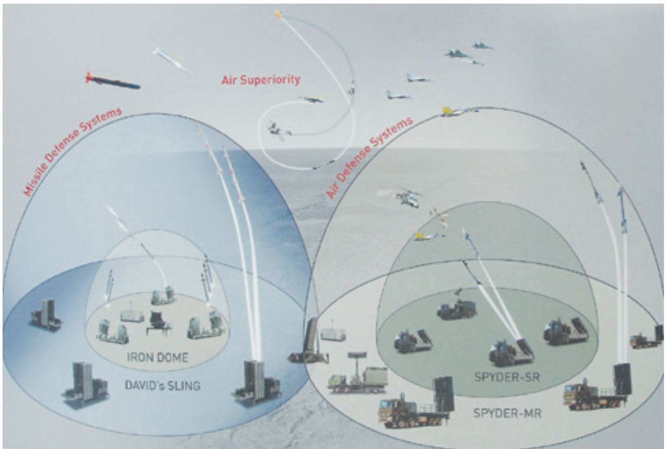
Het principe van de Iron Dome
